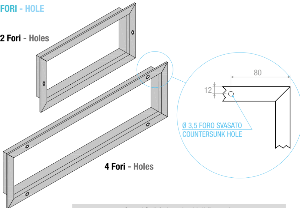
Quantità di fori per le viti di fissaggio Amount of holes for mounting screw
